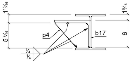
Section AF - AF
